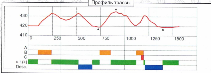
Профиль трассы
