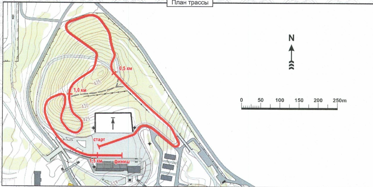
План трассы
