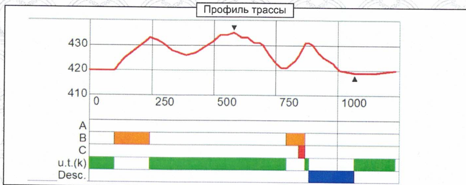
Профиль трассы
