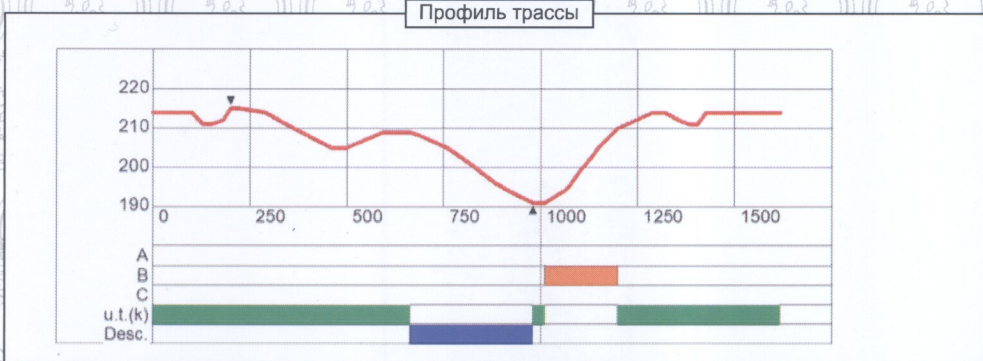
Профиль трассы
