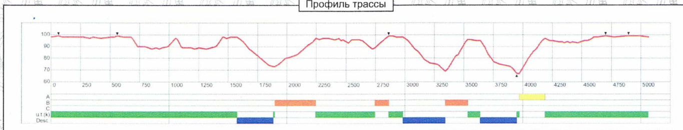
Профиль трассы
