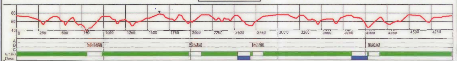
Профиль трассы
