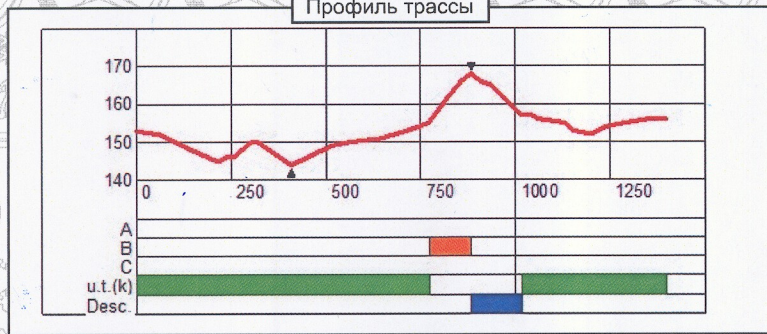
Профиль трассы
