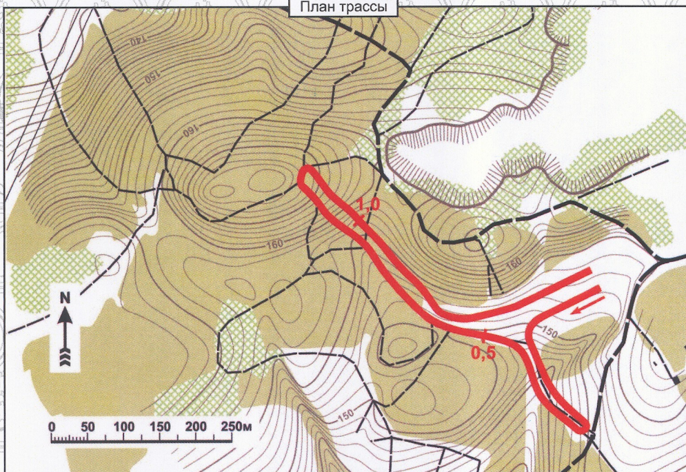
План трассы
