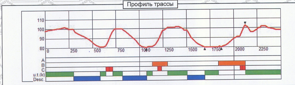
Профиль трассы
