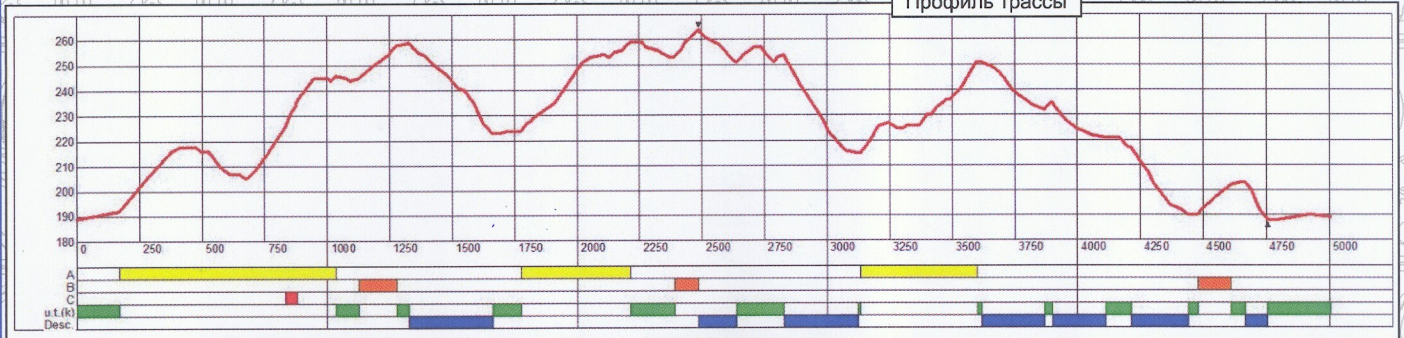
Профиль трассы
