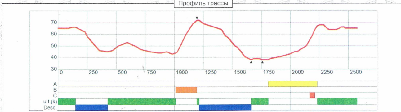
Профиль трассы
