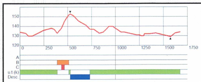
Профиль трассы
