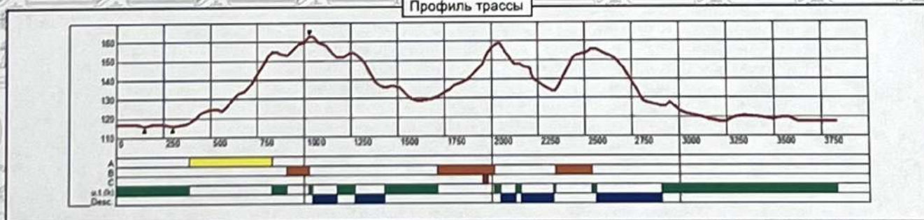
Профиль трассы
