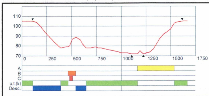
Профиль трассы
