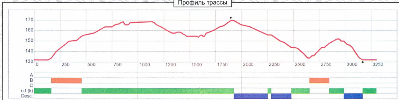
Профиль трассы
