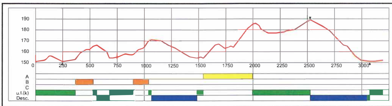
Профиль трассы
