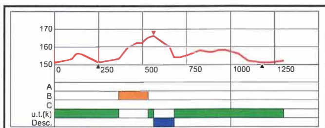
Профиль трассы
