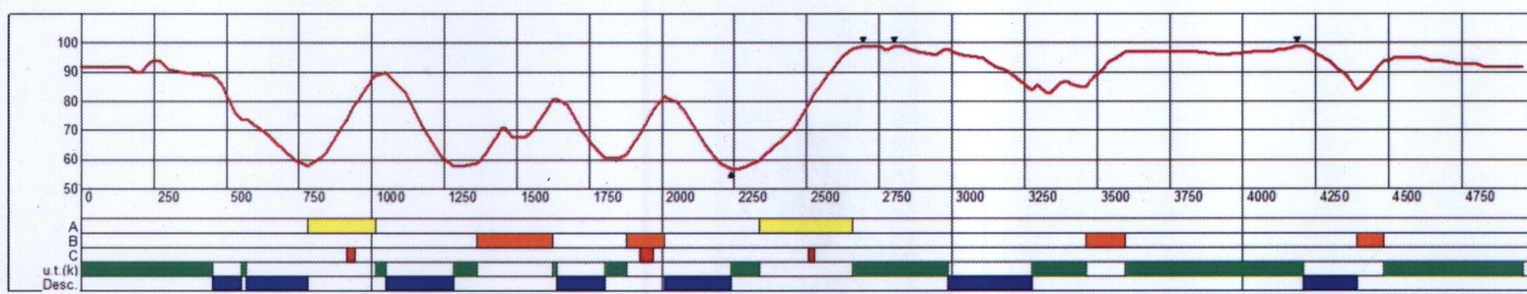
Профиль трассы
