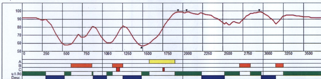
Профиль трассы
