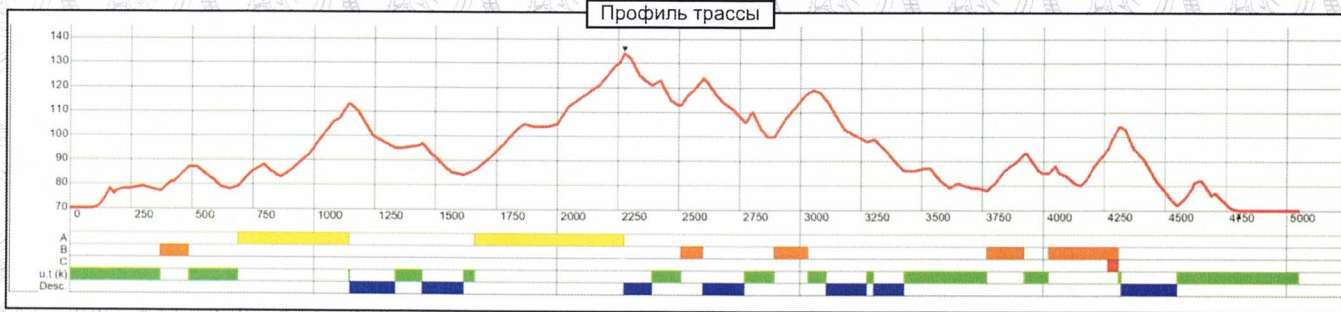
Профиль трассы
