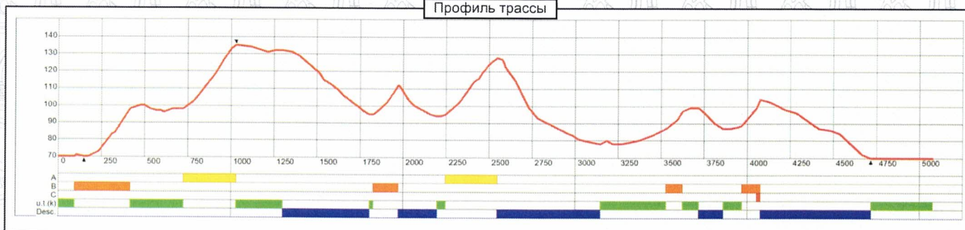
Профиль трассы
