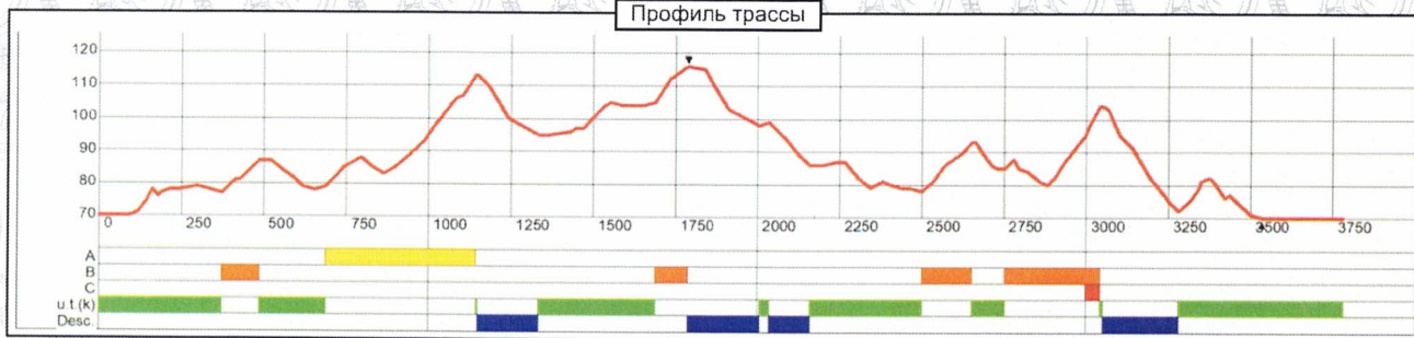
Профиль трассы
