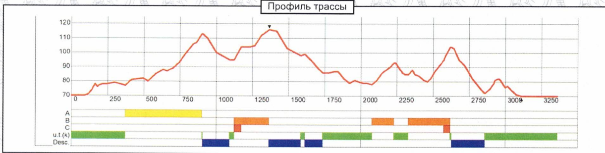
Профиль трассы
