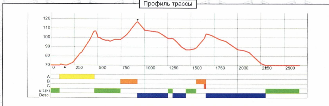
Профиль трассы
