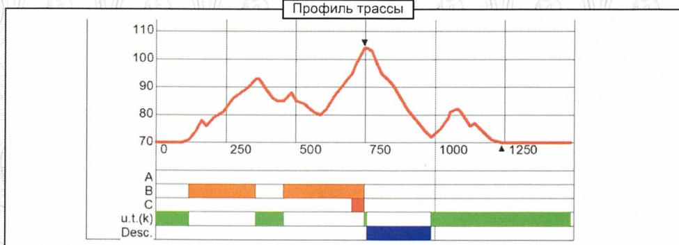
Профиль трассы
