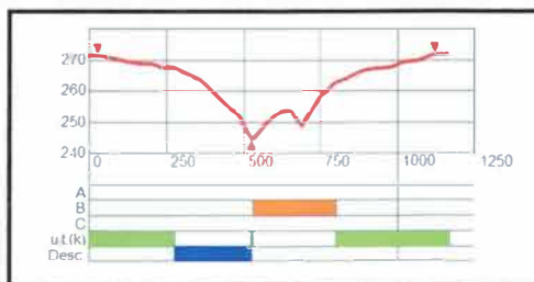
Профиль трассы
