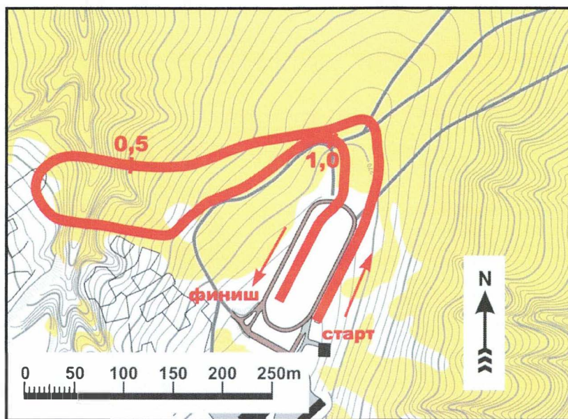
План трассы
