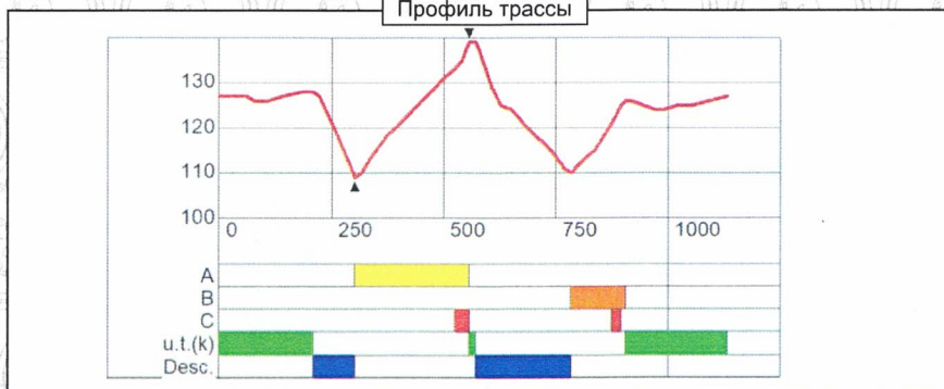
Профиль трассы
