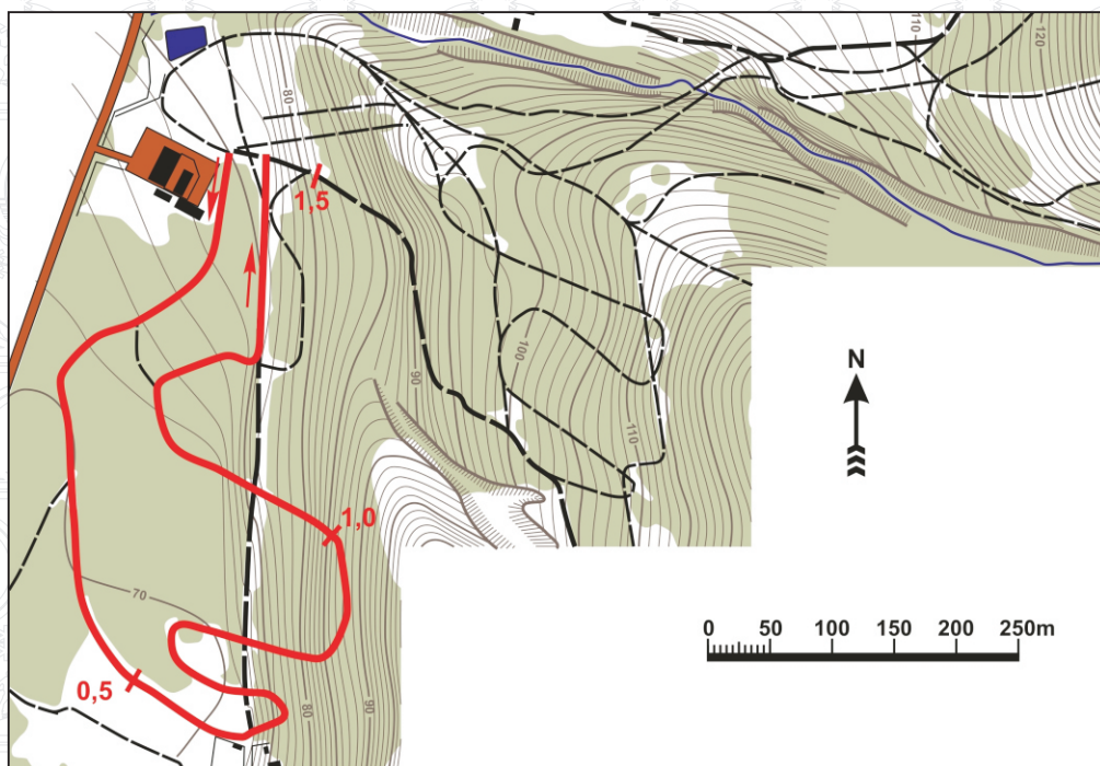
План трассы
