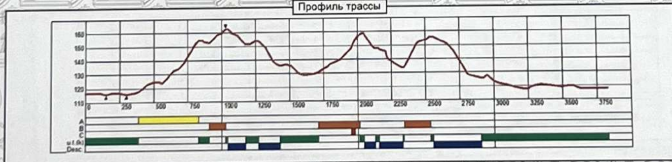
Профиль трассы
