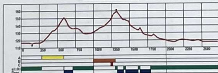
Профиль трассы
